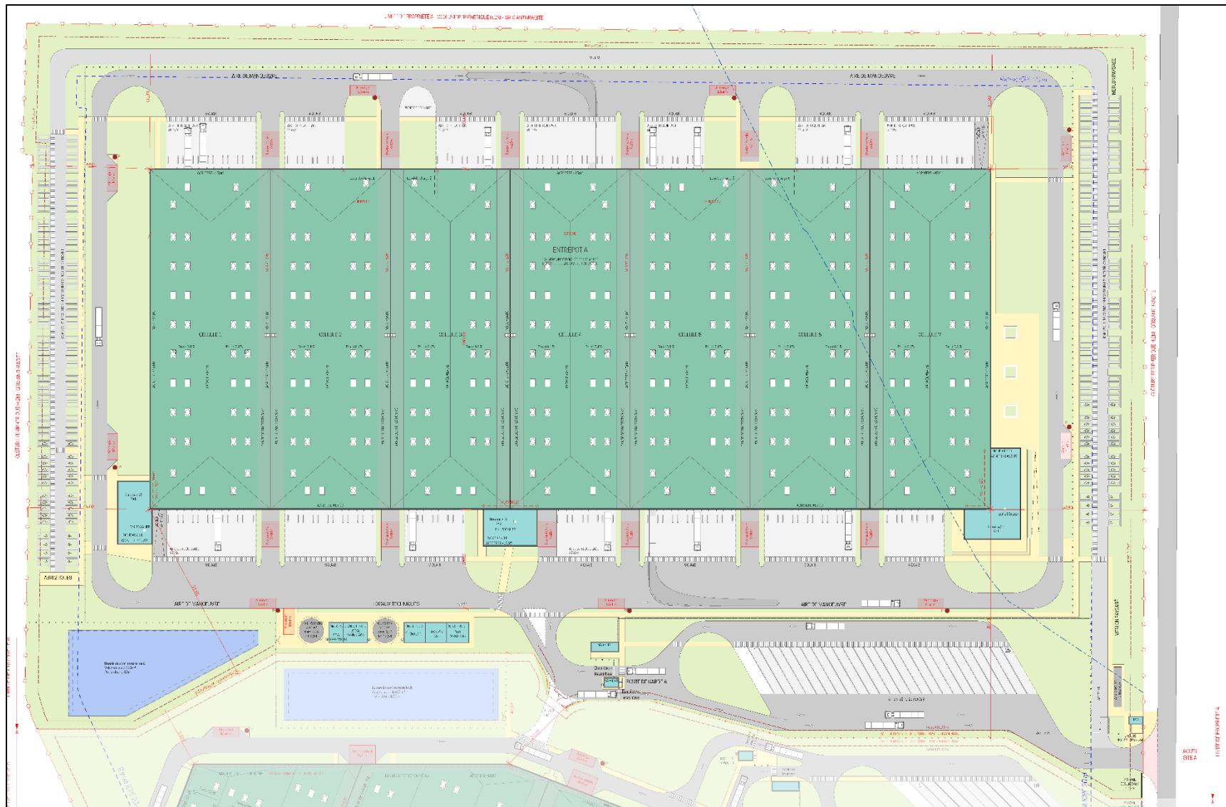
Figure 1 Plan du projet de CATELLA - Bâtiment A
